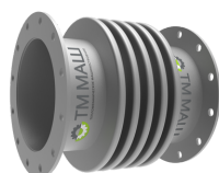
Сильфонные компенсаторы для газоходов (ТММ-КСО)
